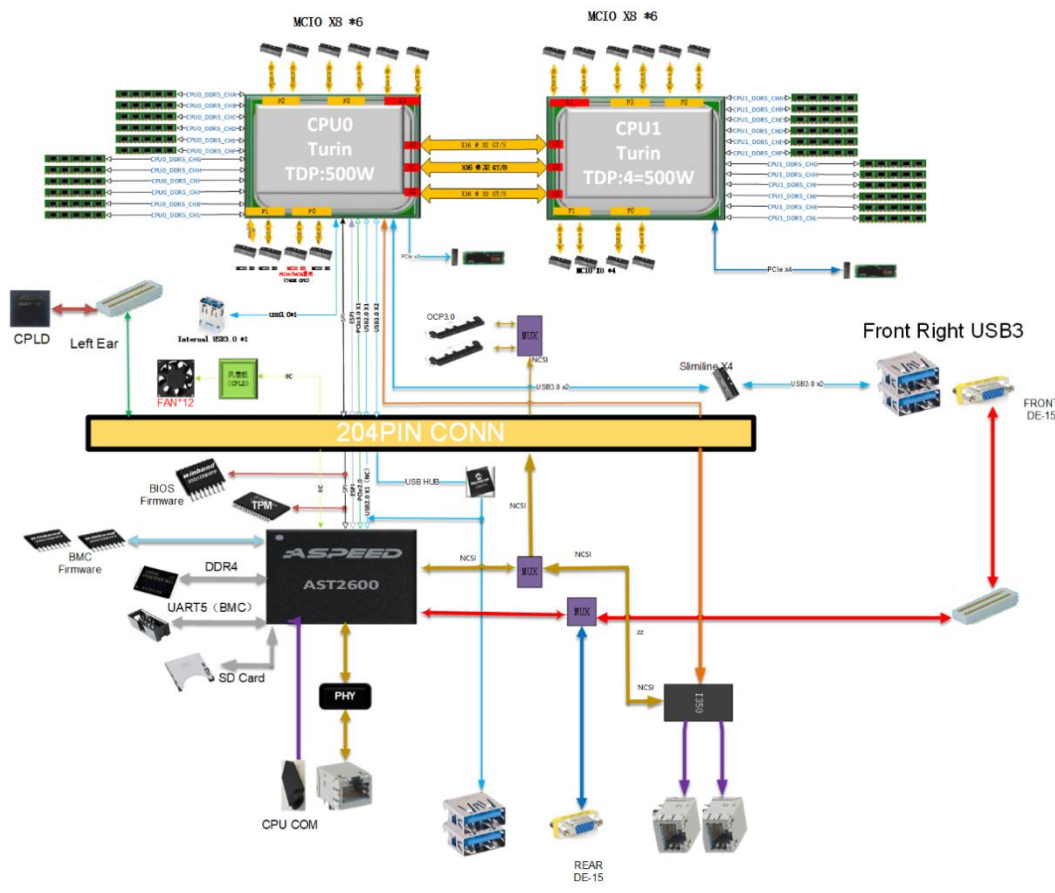
主板逻辑框图
