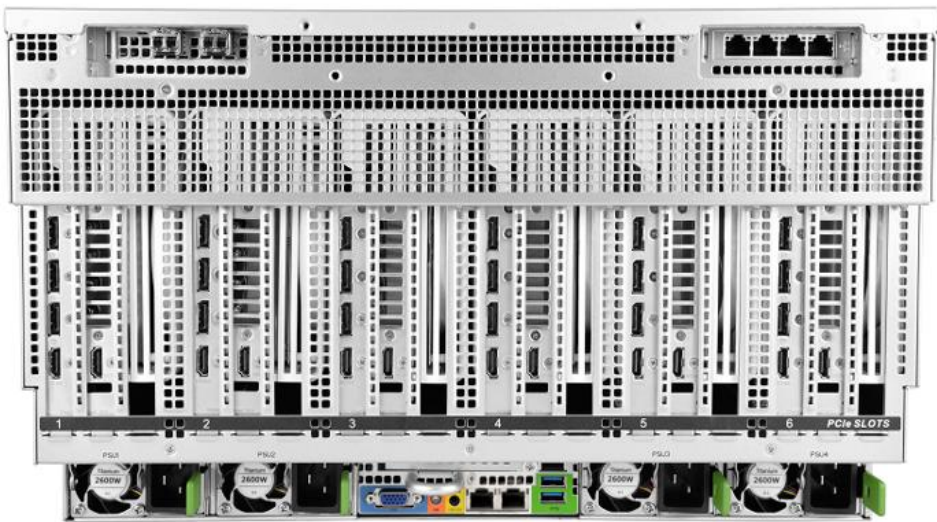
后视图
