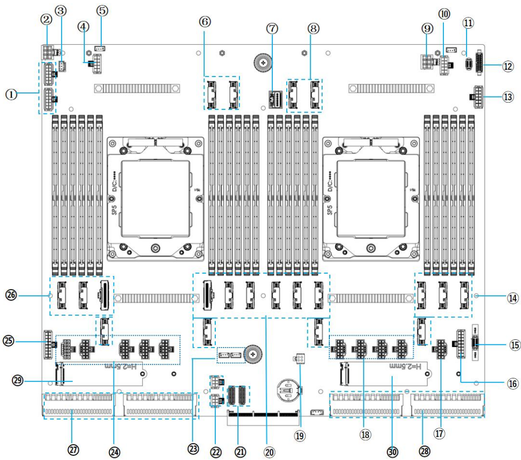
主板图 2-16
